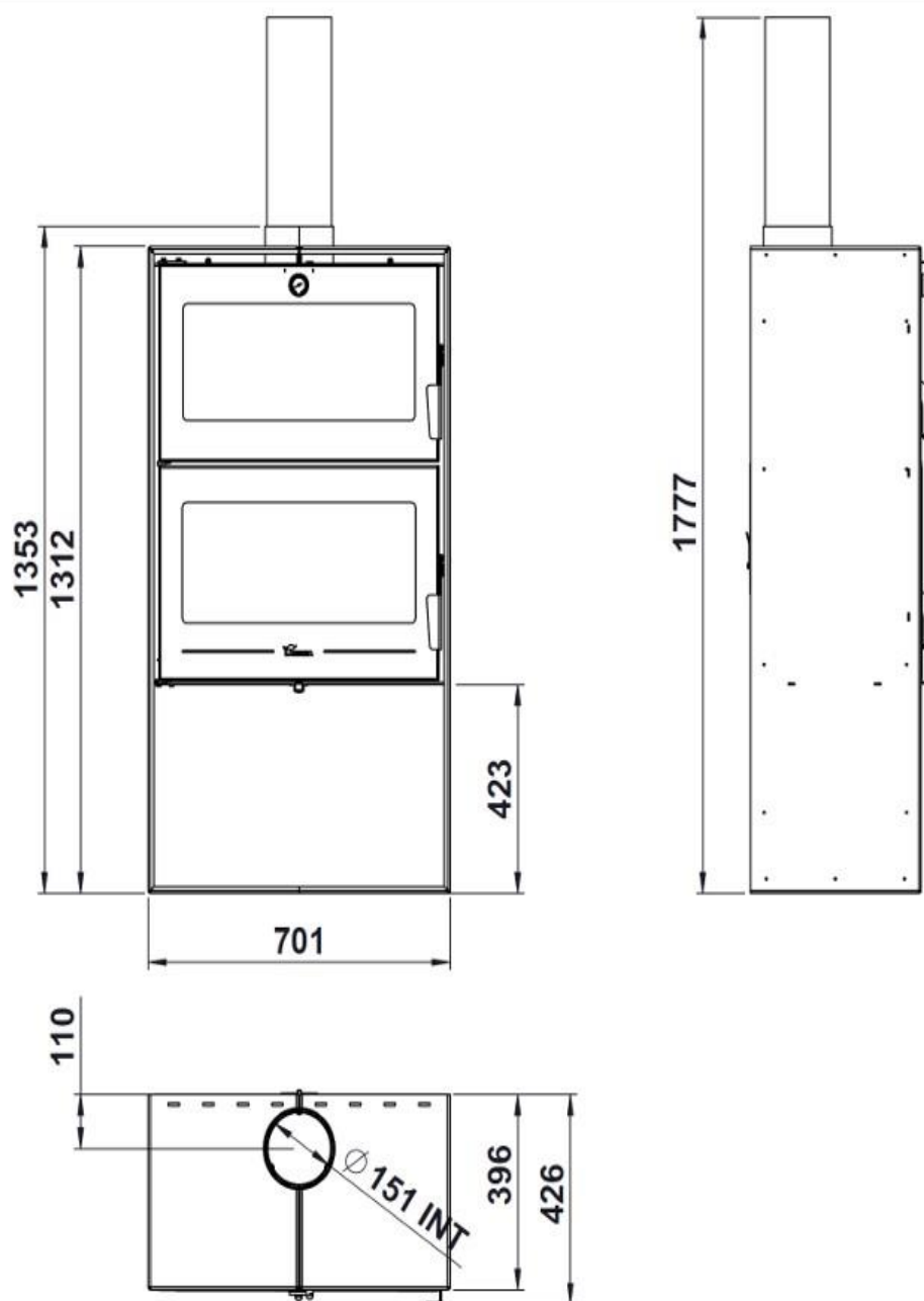
Figura n°1 - Dimensioni in mm dell'apparecchio OSLO
